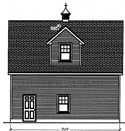
Right Elevation
